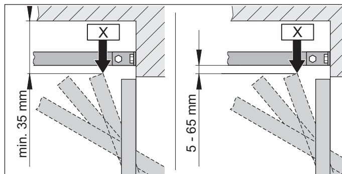
III. 1.1 Point le plus élevé des portes pivotantes et basculantes
