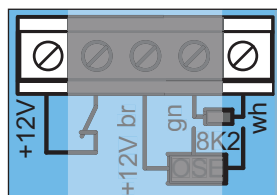
III. Sortie 12 V
