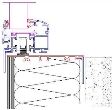
POSE EN NEUF sans habillage
