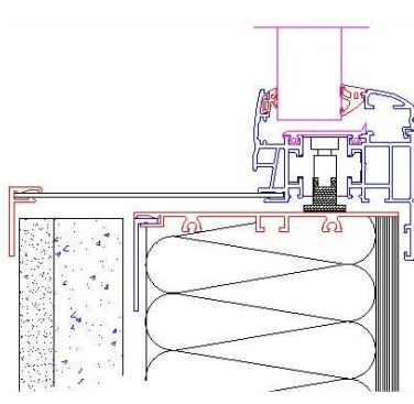
POSE EN NEUF avec habillage
