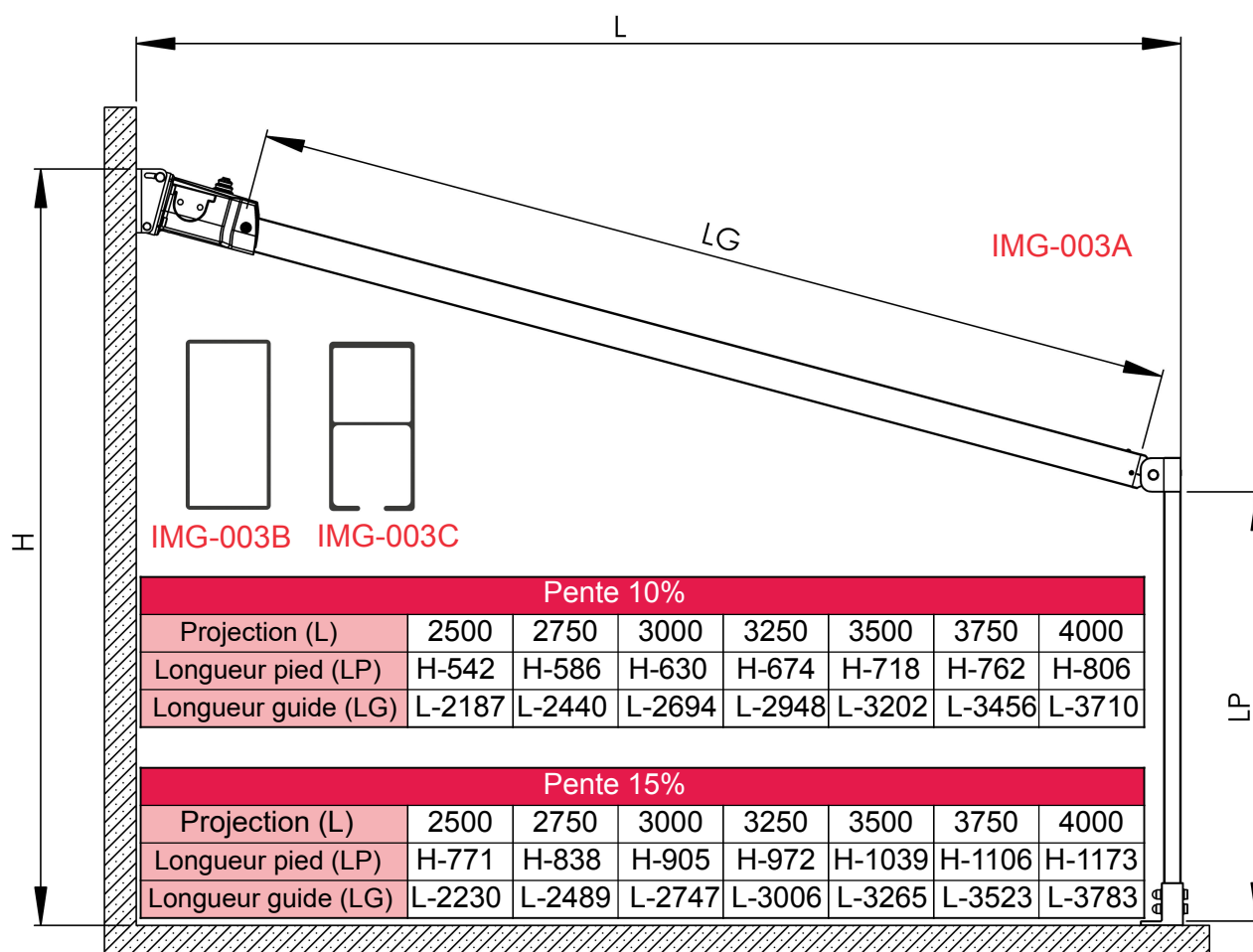
Schéma d'un module simple
