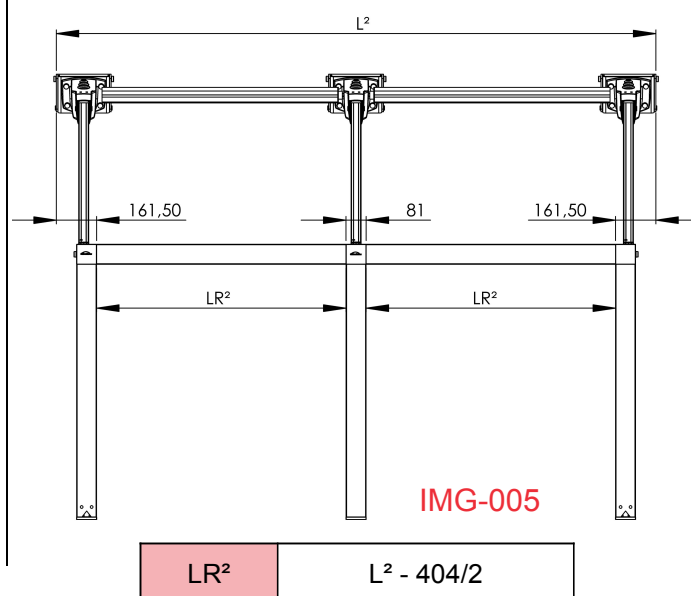
Schéma d'un module double
