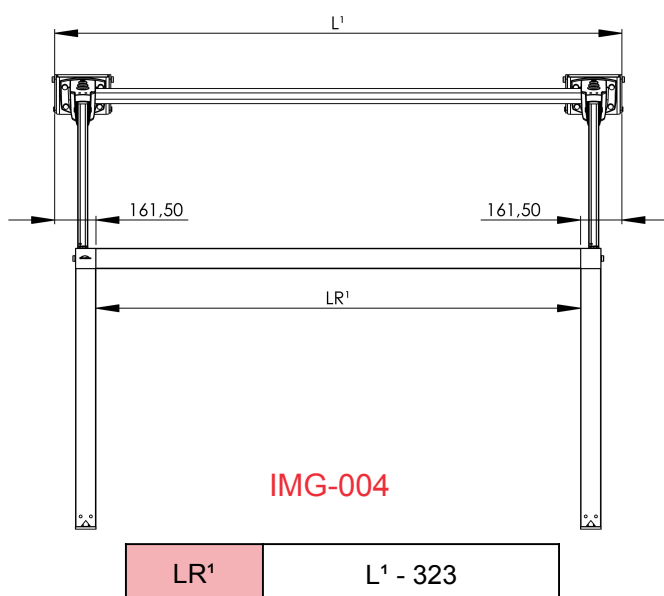
Schéma d'un module simple
