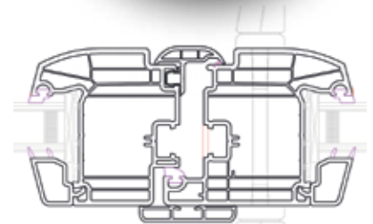
Porte-Fenêtre serrure
