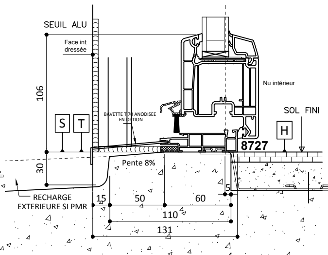
DOUBLAGE DE 160mm
