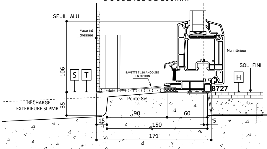
DOUBLAGE DE 160mm
