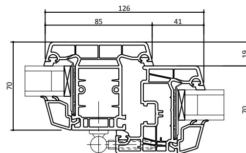
COUPE HORIZONTAL SUR MONTANTS INTERMEDIAIRES OUVRANT + FIXE
