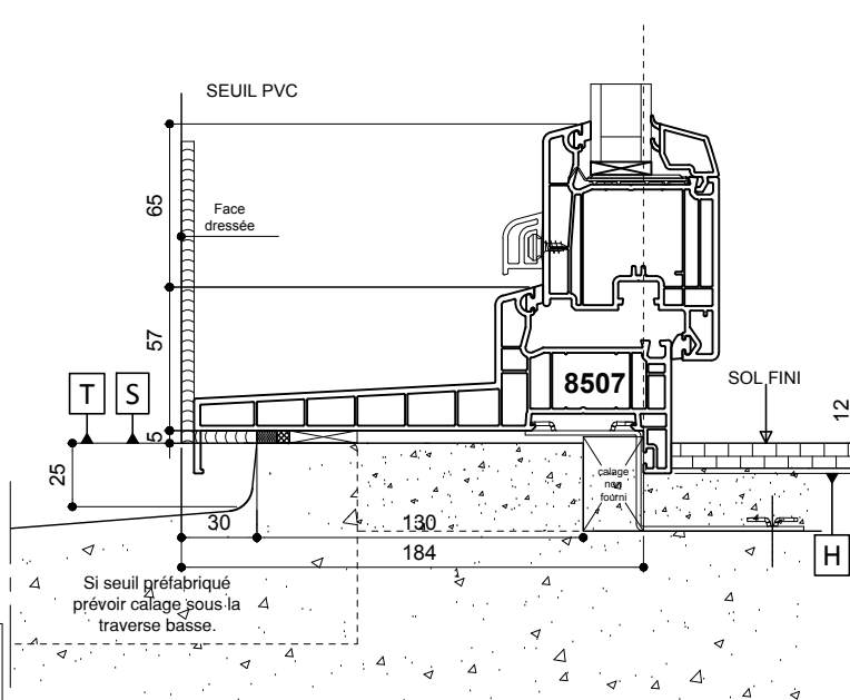
Traverse Basse Porte-Fenêtre
