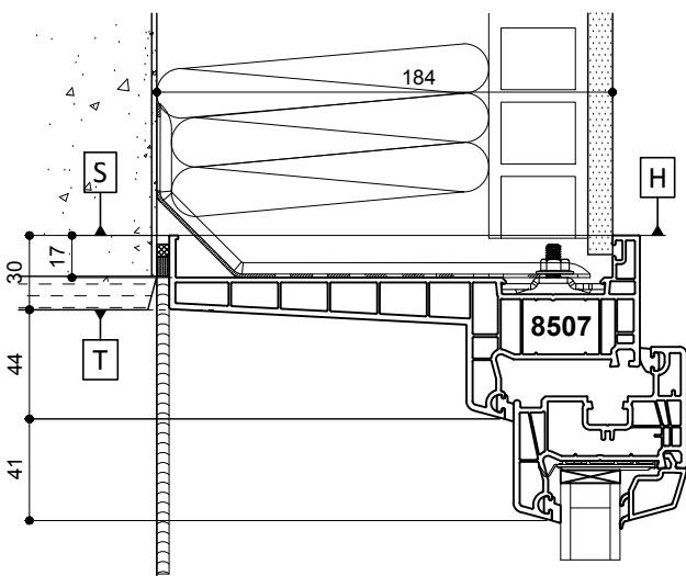
Traverse Basse Fenêtre
