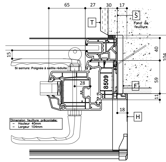
Traverse Basse Porte-Fenêtre avec Seuil ALU plat
