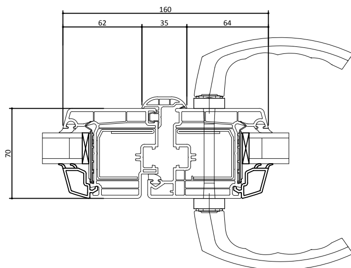
COUPE HORIZONTAL SUR MONTANTS CENTRAUX D'OUVRANTS DE PORTE-FENETRE SERRURE
