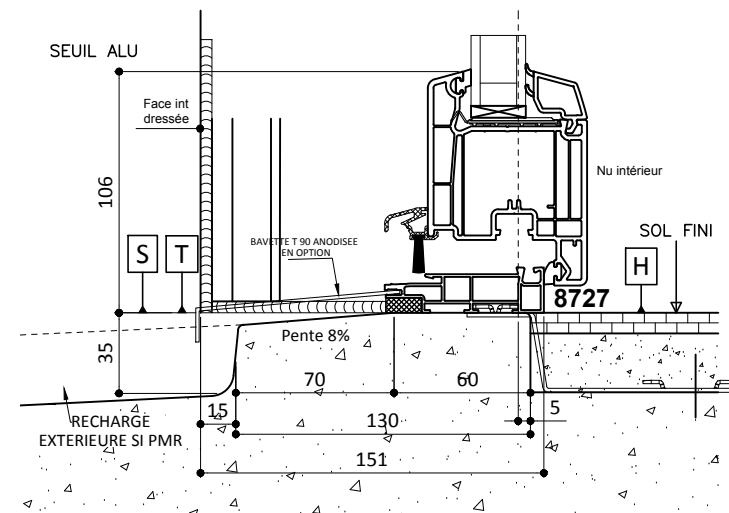
DOUBLAGE DE 180mm
