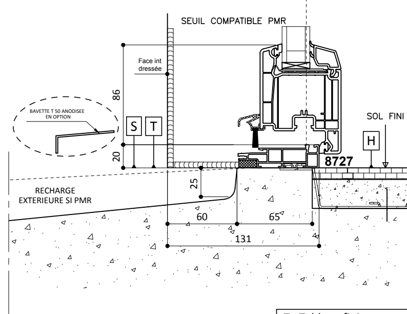
Traverse Basse Porte-Fenêtre avec Seuil ALU plat
