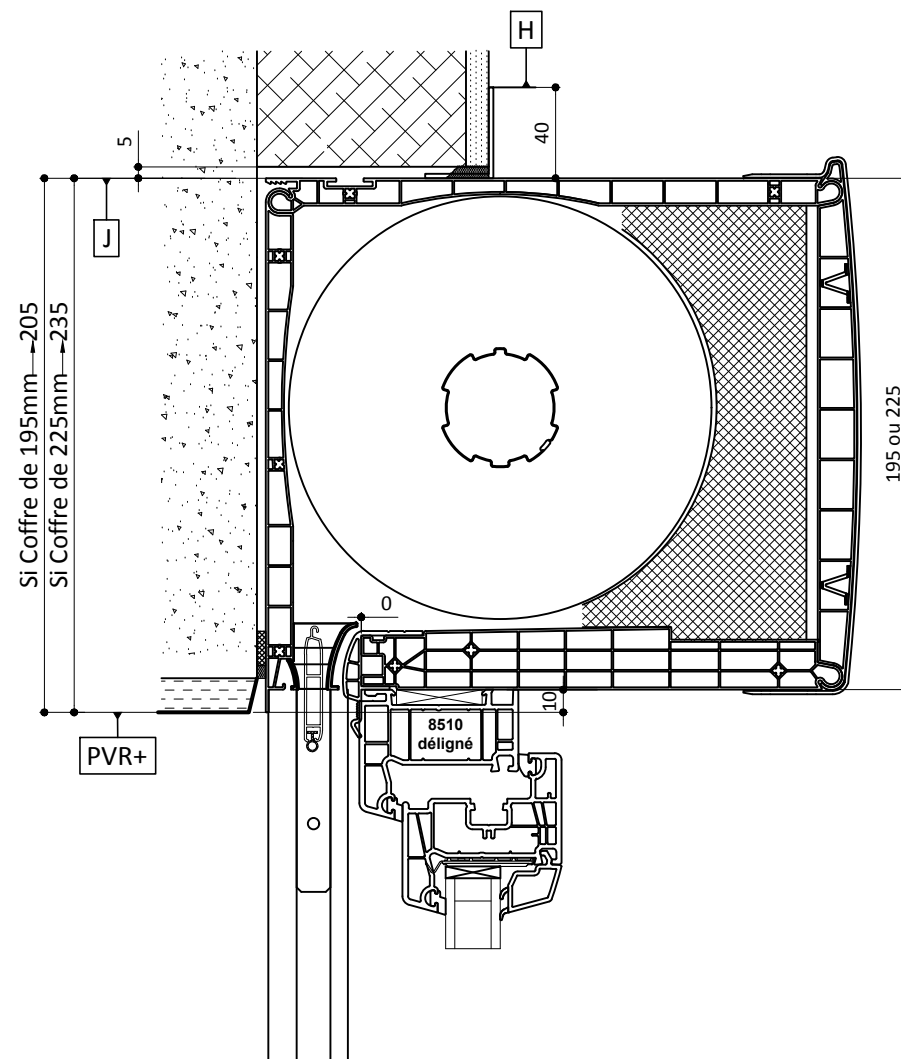
Dépose de la traverse haute
