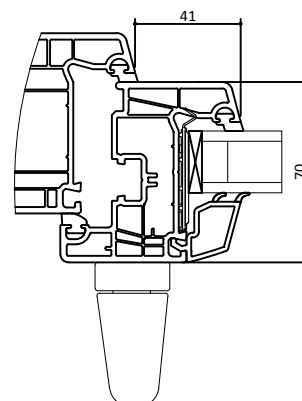
COUPE HORIZONTAL SUR MONTANTS LATERAUX D'OUVRANTS DE FENETRE ET DE PORTE-FENETRE
