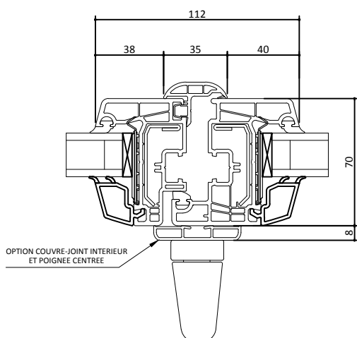
COUPE HORIZONTAL SUR MONTANTS CENTRAUX D'OUVRANTS DE FENETRES ET DE PORTES-FENETRES
