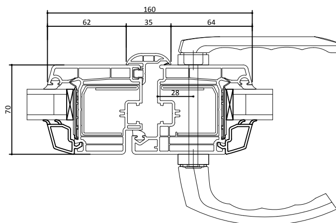
COUPE HORIZONTAL SUR MONTANTS CENTRAUX D'OUVRANTS DE PORTE FENETRE SERRURE POIGNEE A SALLIE REDUITE
