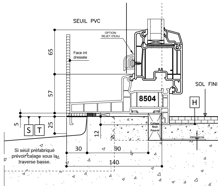
Traverse Basse Porte-Fenêtre
