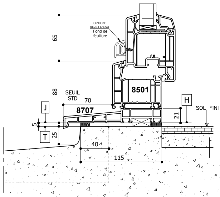
Traverse Basse Porte-Fenêtre
