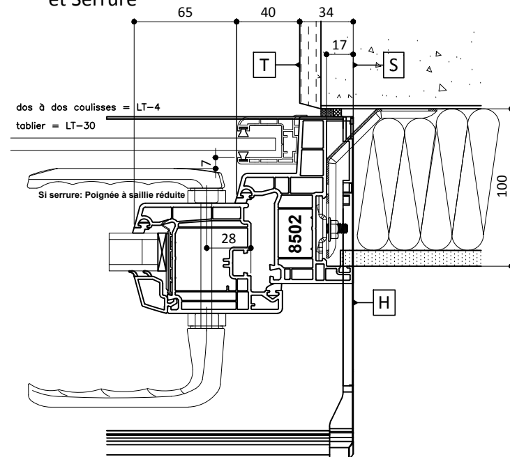
Montant avec Volet Roulante EVIBAIE (Monobloc) et Serrure
