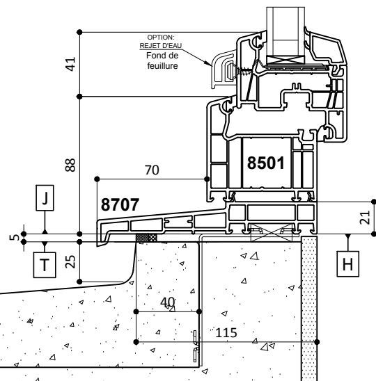
Traverse Basse Fenêtre
