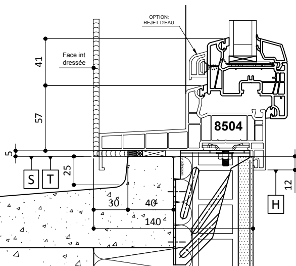
Traverse Basse Fenêtre
