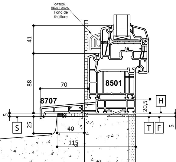
Traverse Basse Fenêtre
