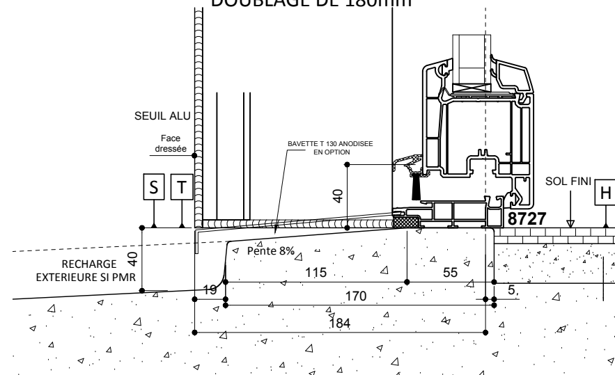
DOUBLAGE DE 180mm
