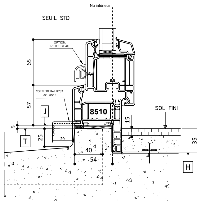
Traverse Basse Porte-Fenêtre
