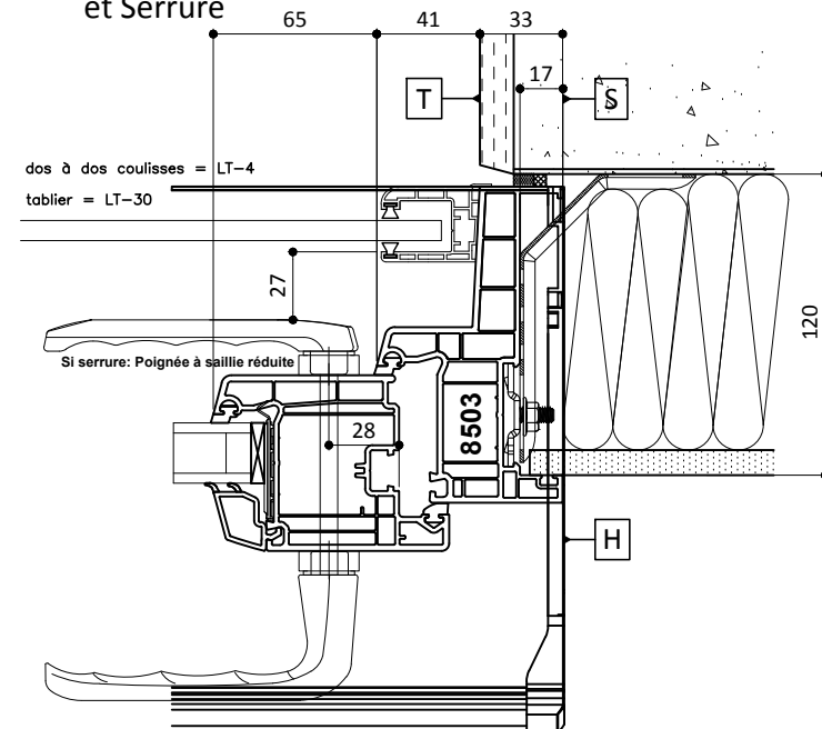
Montant avec Volet Roulant EVIBAIE (Monobloc) et Serrure
