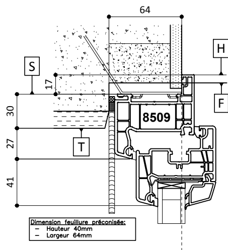
Traverse Basse Fenêtre
