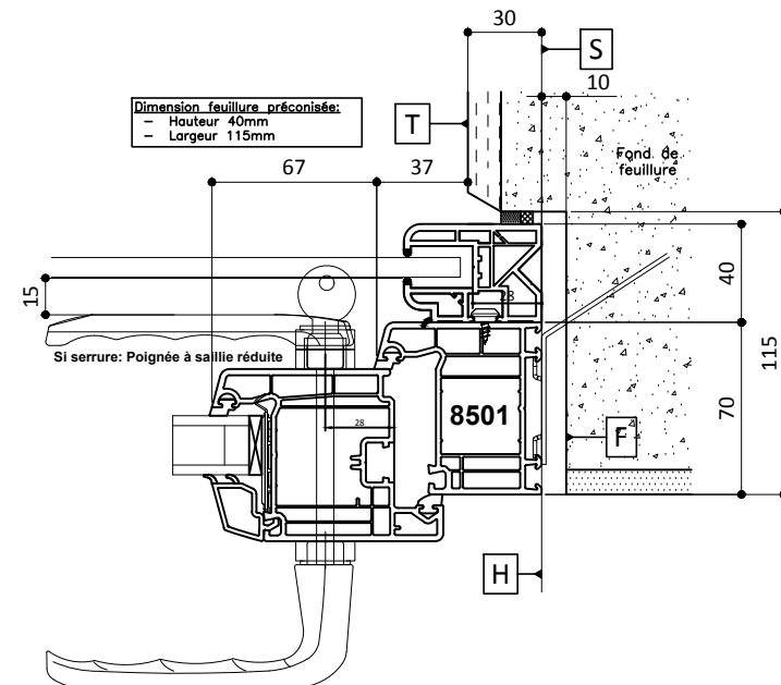
Traverse Basse Porte-Fenêtre avec Seuil ALU plat
