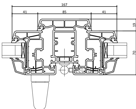
COUPE HORIZONTAL SUR MONTANTS INTERMEDIAIRES OUVRANT + OUVRANT
