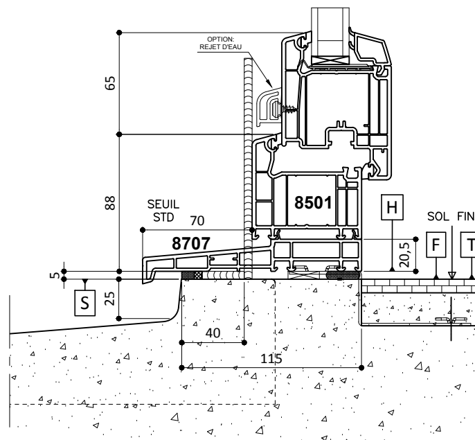
Traverse Basse Porte-Fenêtre
