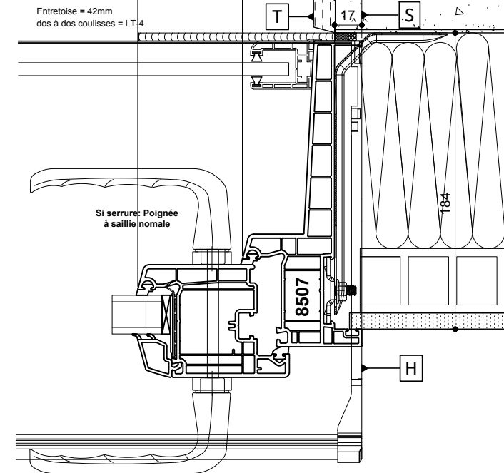
Montant avec Volet Roulant EVIBAIE (Monobloc) et Serrure
