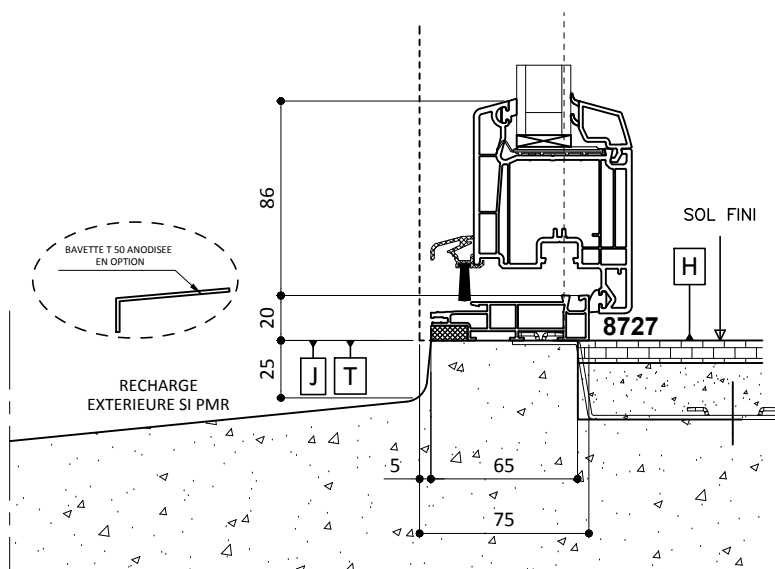
Traverse Basse Porte-Fenêtre avec Seuil ALU plat
