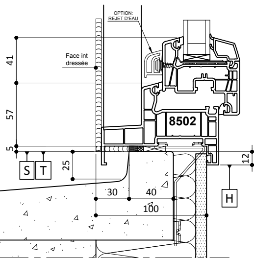
Traverse Basse Fenêtre
