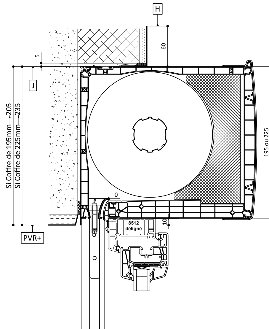
Dépose de la traverse haute
